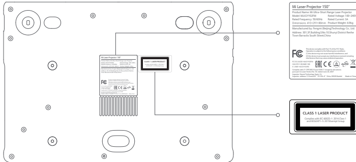
Plaque signalétique du Mi Laser Projector 150 o
