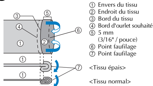
<Vu de côté>
