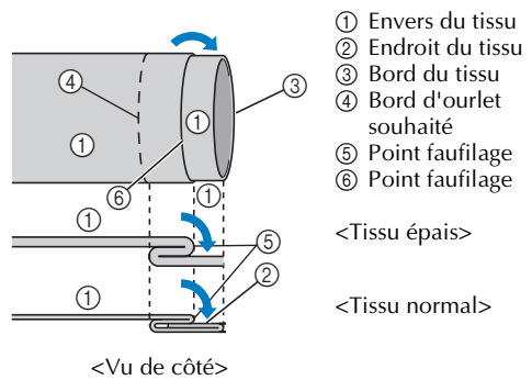
<Vu de côté>
